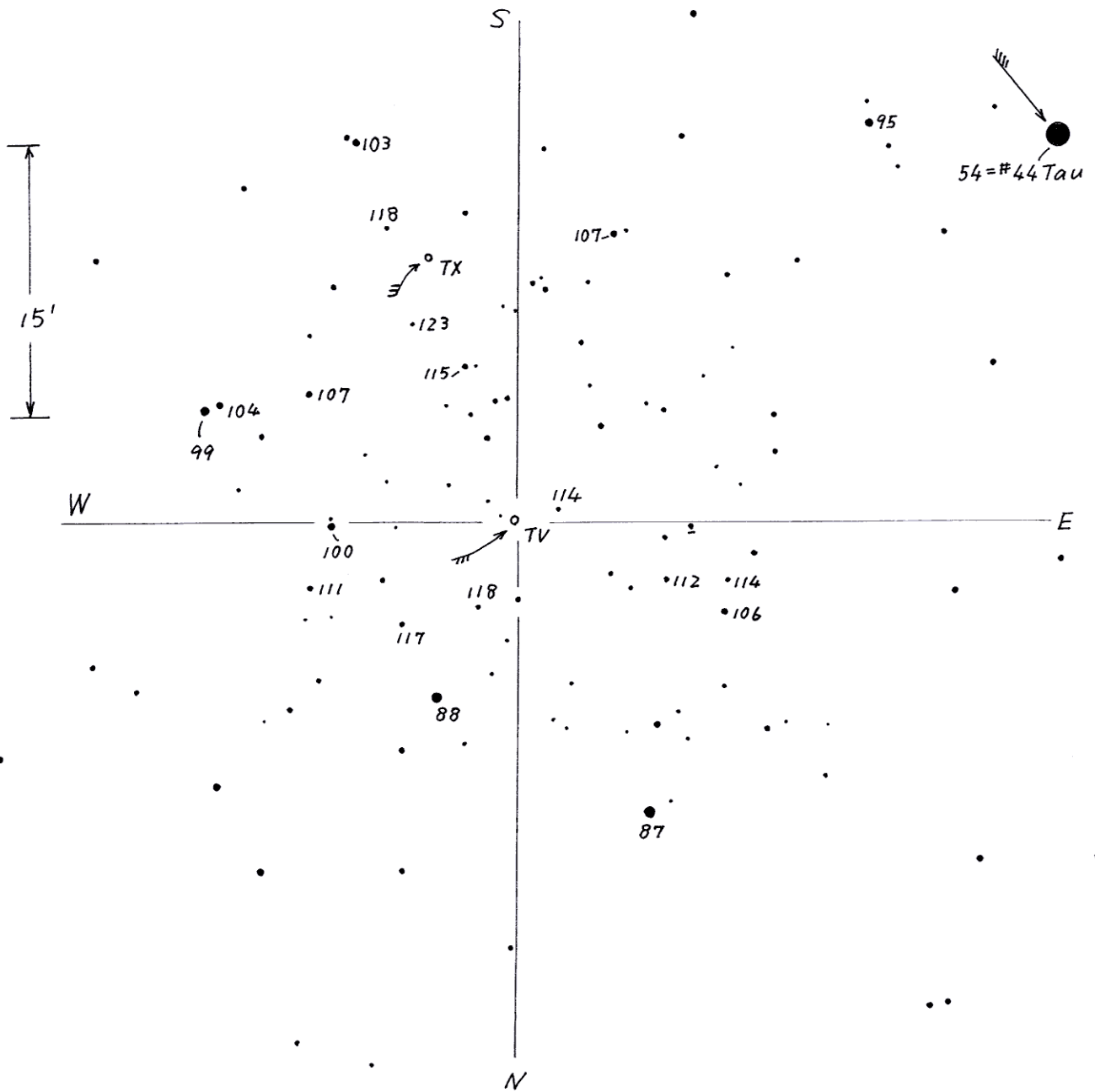
AAVSO (d) Chart
