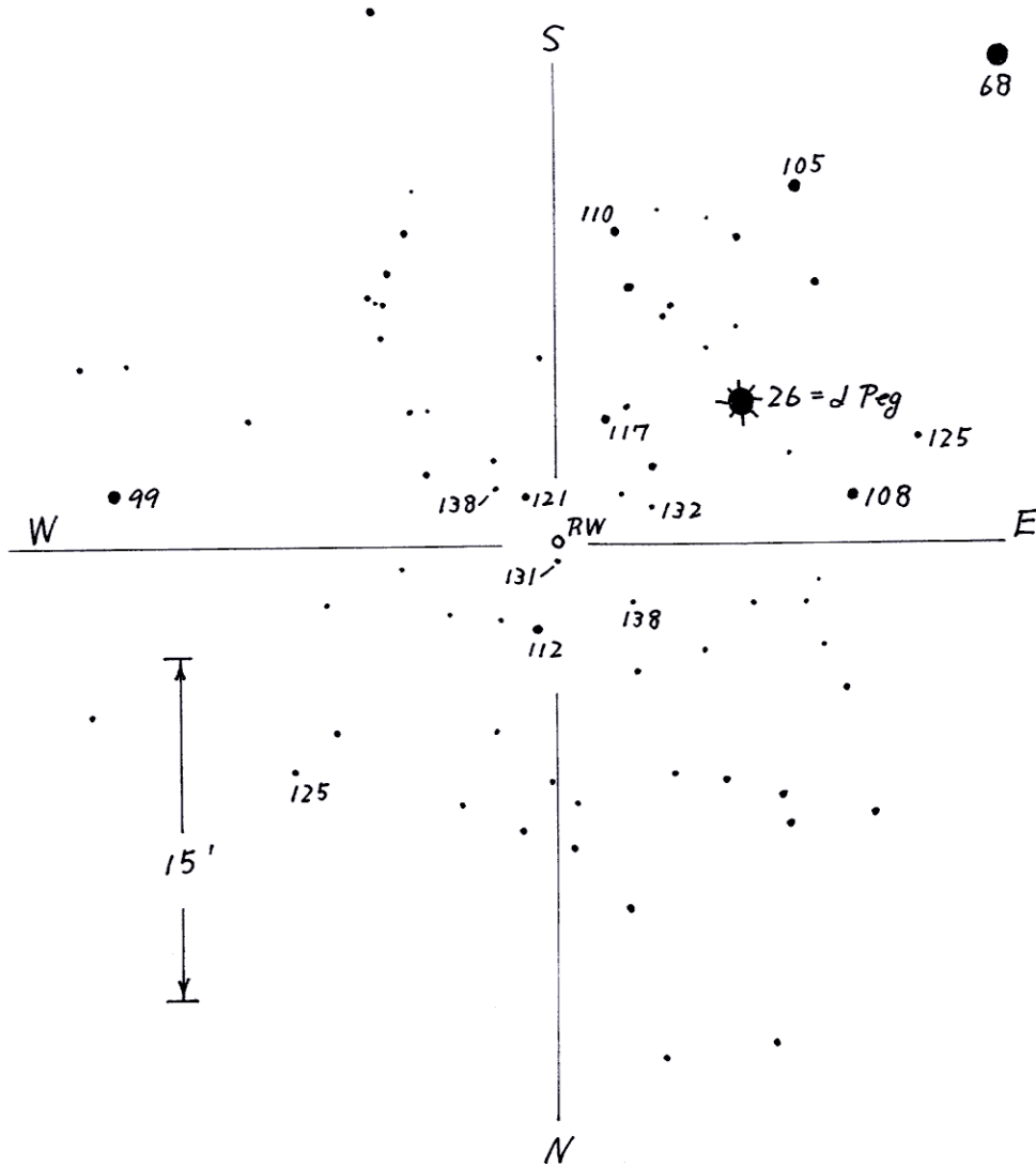
AAVSO (d) Chart
