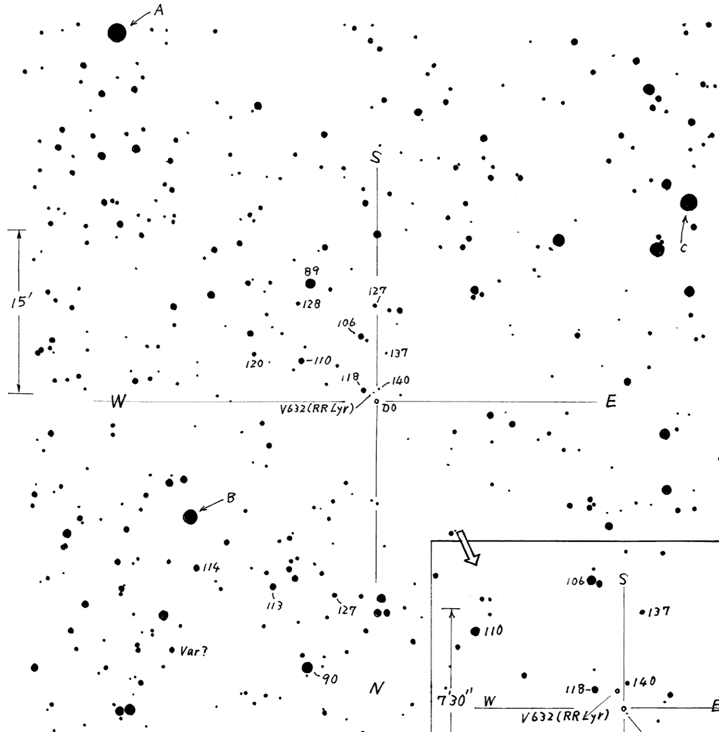
AAVSO (d) chart
