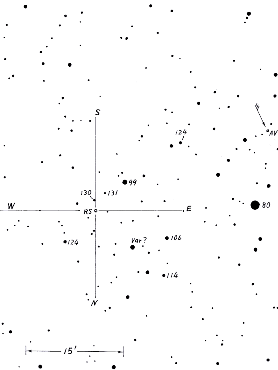
AAVSO (d) Chart
